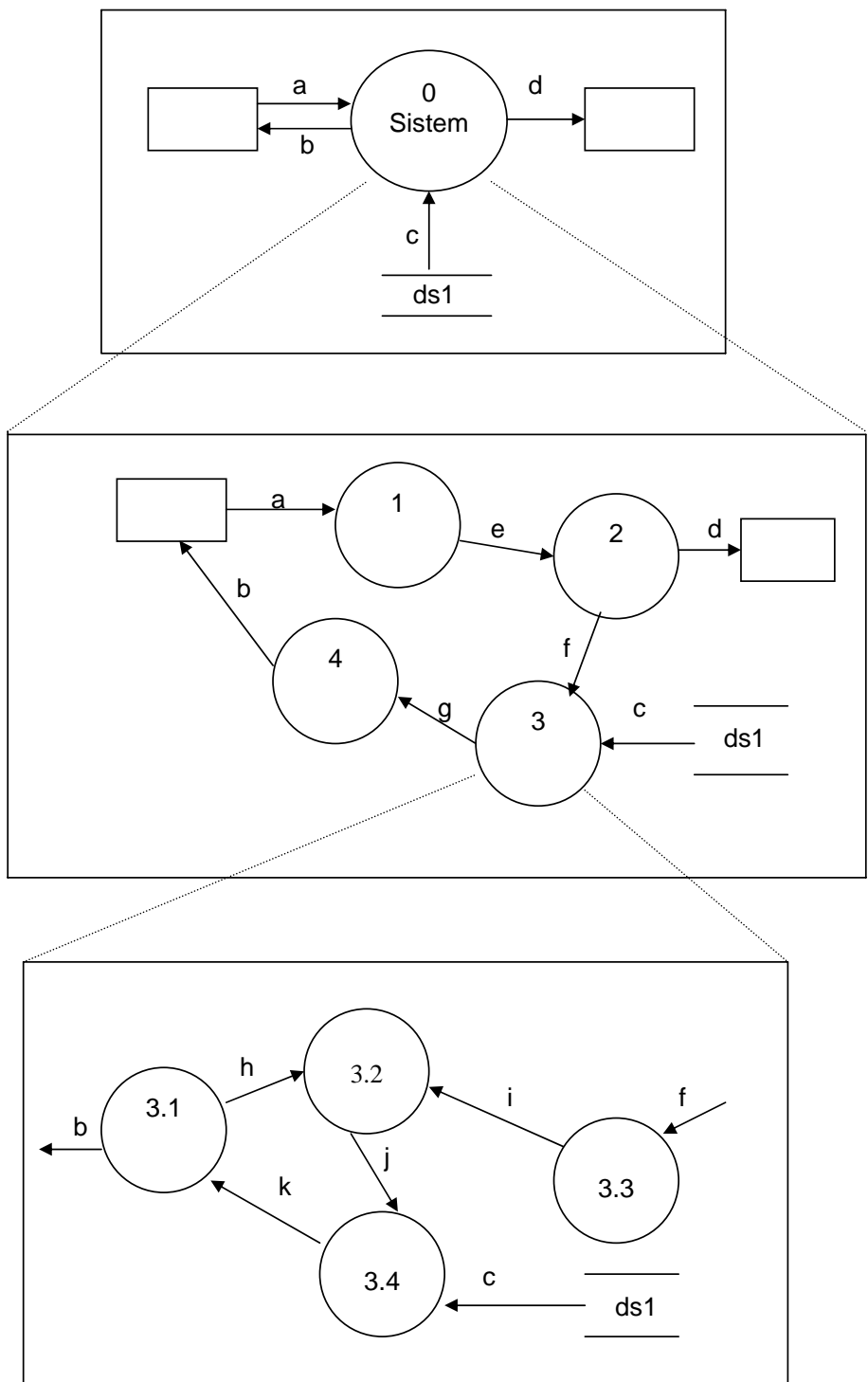
Gambar 11. Levelisasi DFD
