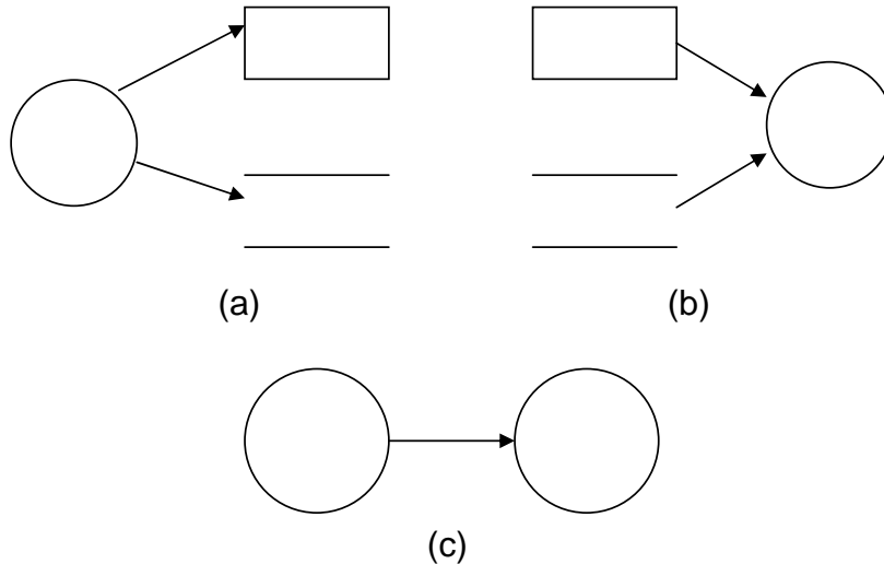
Gambar 6. Konsep sumber atau tujuan alur data
